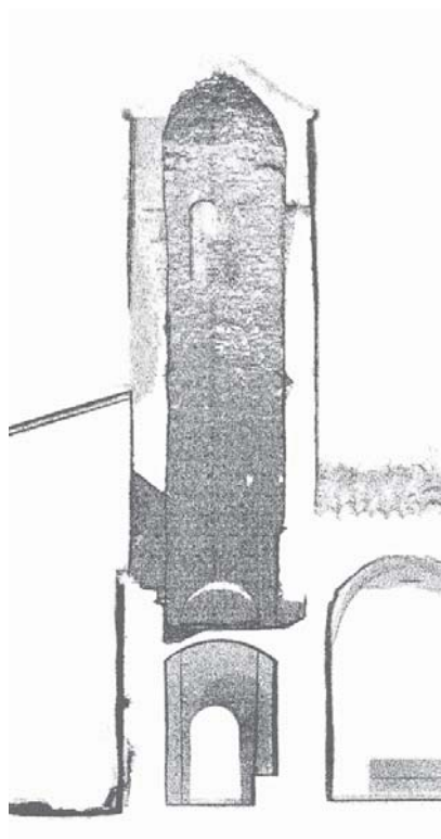
alçat interior campanar mirant al nord
